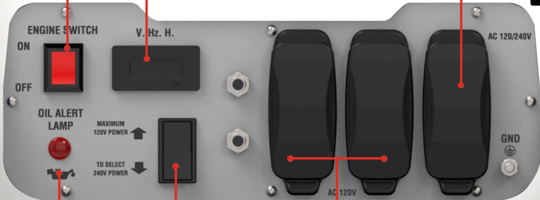
(2) 120V AC 20A 5-20R
